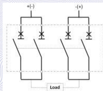
4P 外形接线图 (DC1000V)
