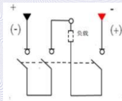
4P 外形接线图 (DC1000V)
